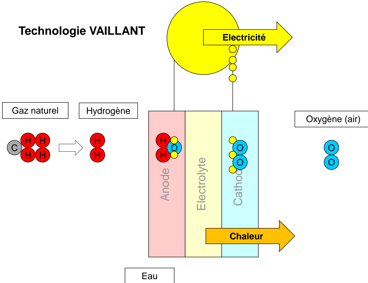
Pile à combustible céramique – SOFC (Solid Oxid Fuel Cell)
